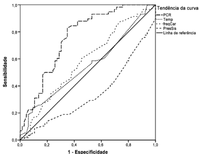
Figura 2. Curva ROC de PCR e variáveis clínicas.
